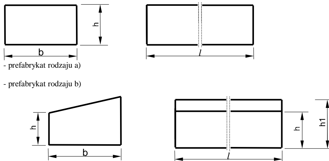
Rys. 7. Wymiarowanie prefabrykatów
